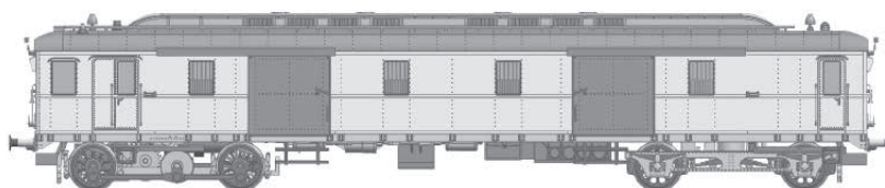
Diesel-Gepäcktriebwagen VT 69 900, DB, Epoche III Diesel baggage railcar VT 69 900, DB, Epoch III
